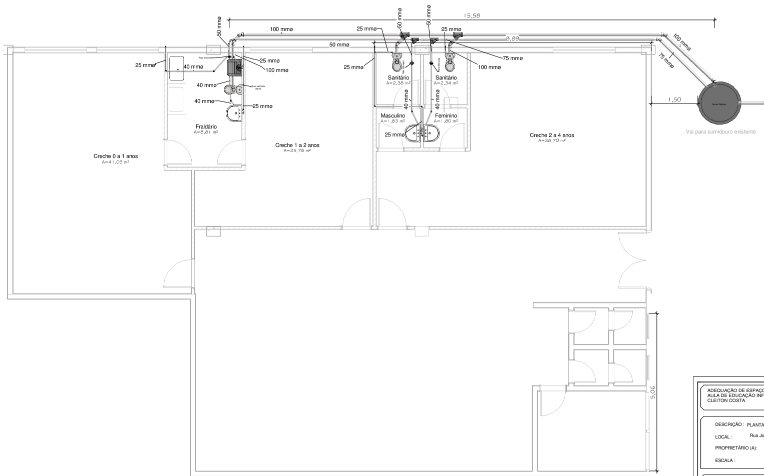
1 Hidrossanitário 1 : 50
